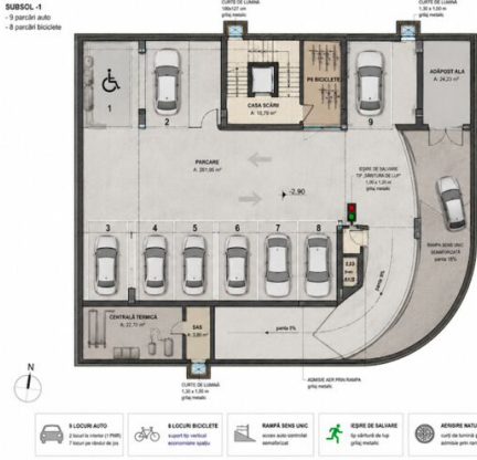
PLAN SUBSOL - PARCĂRI
