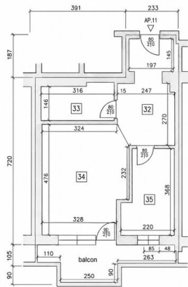
RELEVU APARTAMENT 11 ETAJ 1
